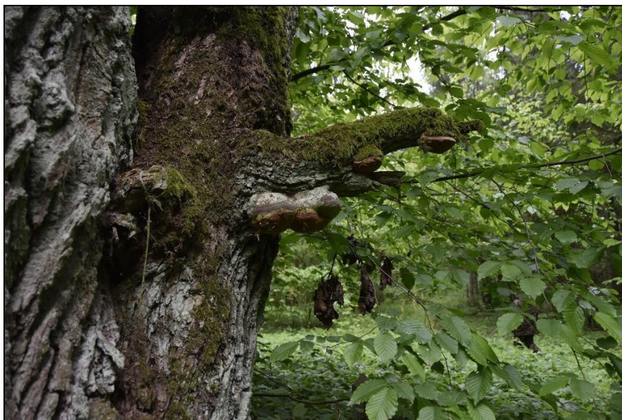
Рисунок 2.3 – Поражение дуба-тройника древесными грибами
