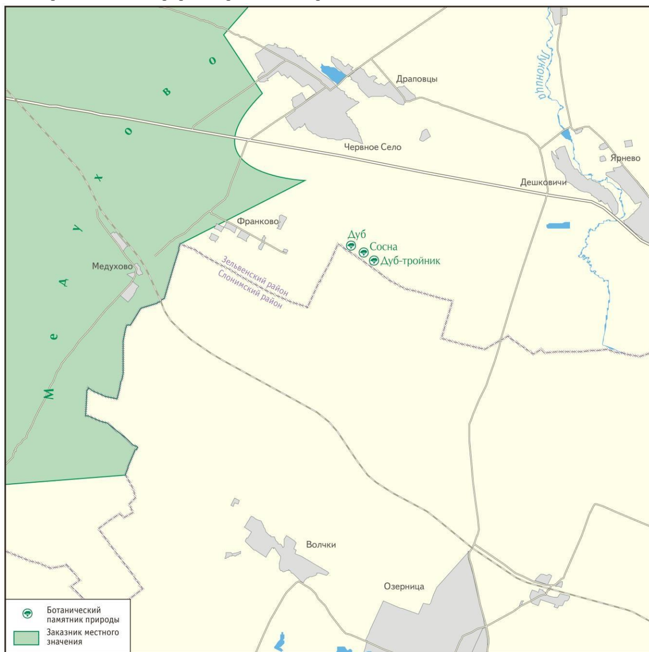
Рисунок 2.1 – Ситуационная схема расположения ботанического памятника природы местного значения «Дуб-тройник»
